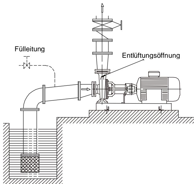
Auffüllung einer Pumpe im Saugbetrieb mit Fußventil
