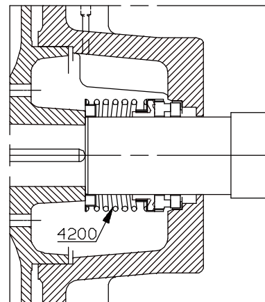
Entlastete Gleitringdichtung
