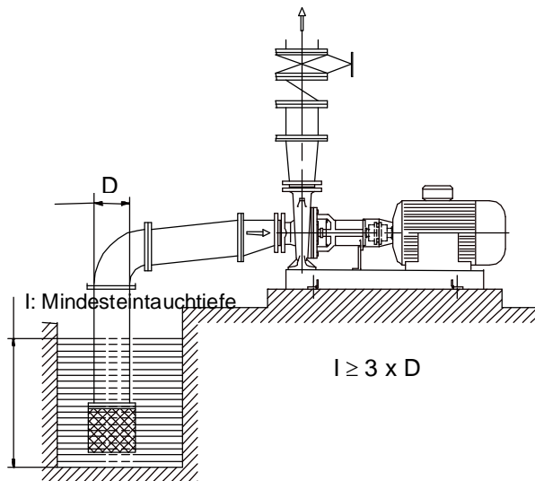
Pumpe im Saugbetrieb
