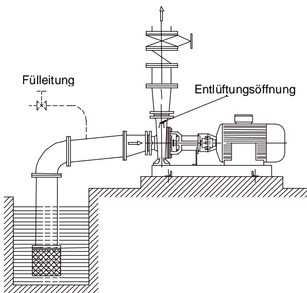
Auffüllung einer Pumpe im Saugbetrieb mit Fußventil
