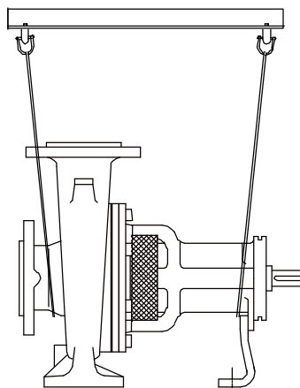
Pumpe allein
