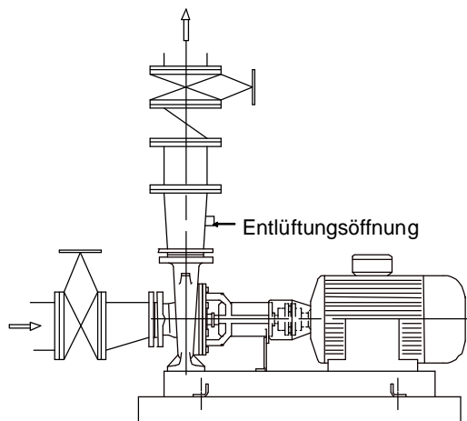
Auffüllen einer Pumpe mit Zulauf
